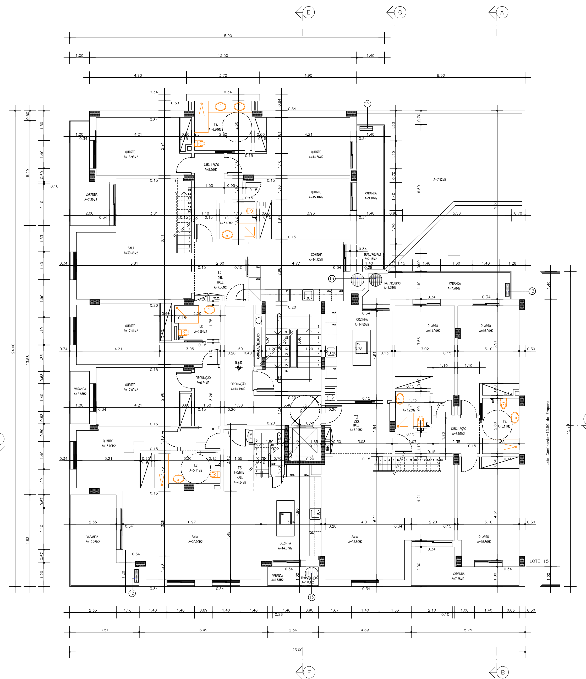
PLANTA PISO 4
